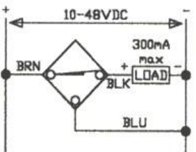
Cable - PNP/N.C. Wiring Diagram #2
